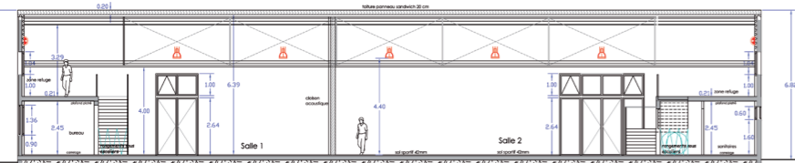
COUPE LONGITUDINALE A A
