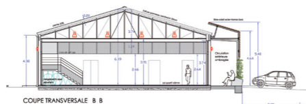
COUPE TRANSVERSALE B B
